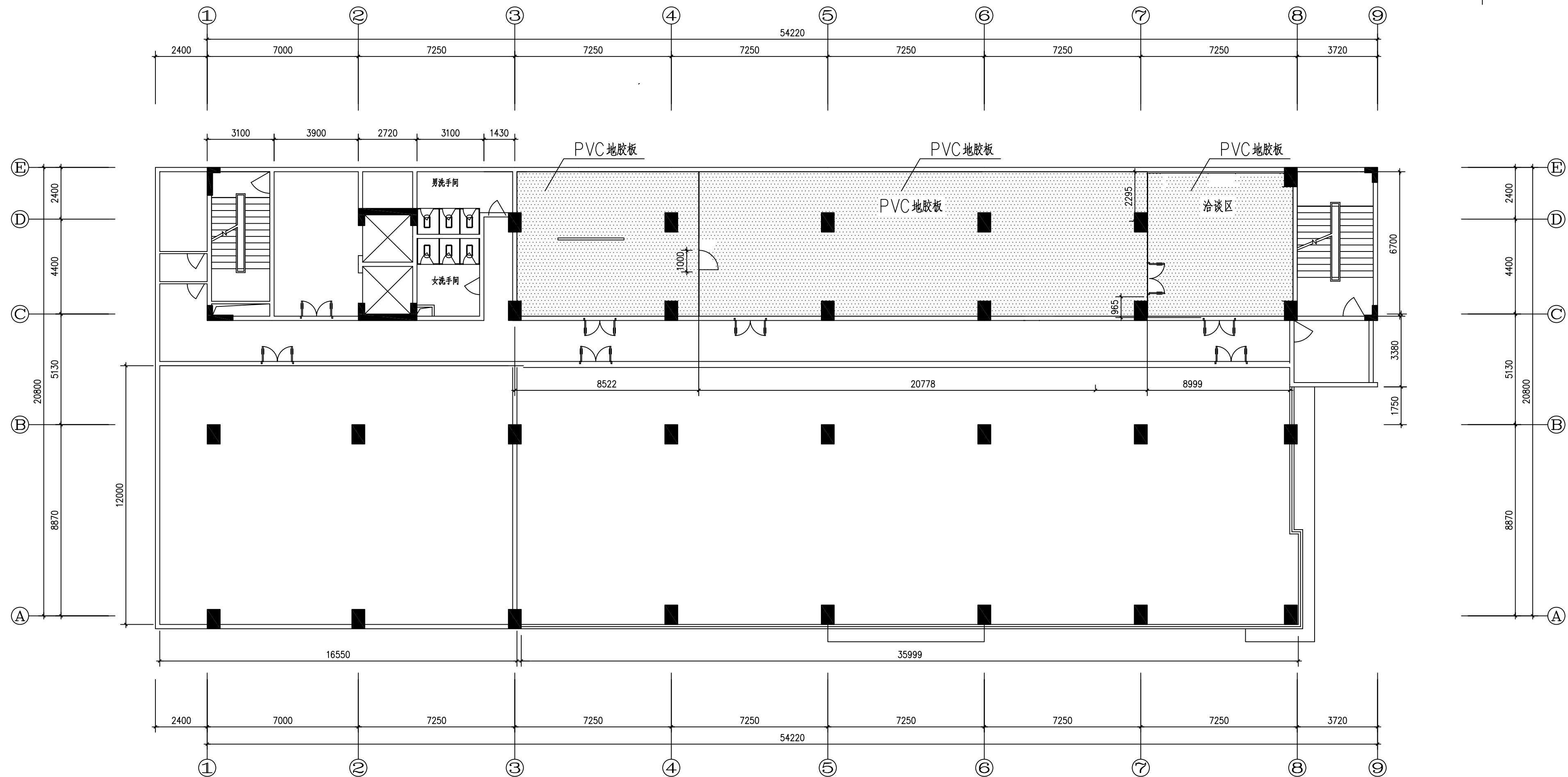
七层地花图 1:100
